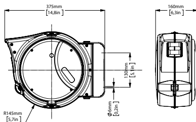
dimensions AM80
